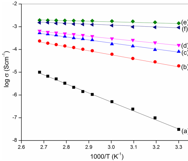
Fig. 7 Arrhenius plot of (a) pure P(VdCl...), (b) 70 wt% P(VdCl...):30 wt% MgCl 2 , (c) 70 wt% P(VdCl...): 30 wt% MgCl 2 : 0.1 wt% SN, (d) 70 wt% P(VdCl...): 30 wt% MgCl 2 : 0.2 wt% SN, (e) 70 wt% P(VdCl...): 30 wt% MgCl 2 : 0.3 wt% SN, (f) 70 wt% P(VdCl...): 30 wt% MgCl 2 : 0.4 wt% SN
