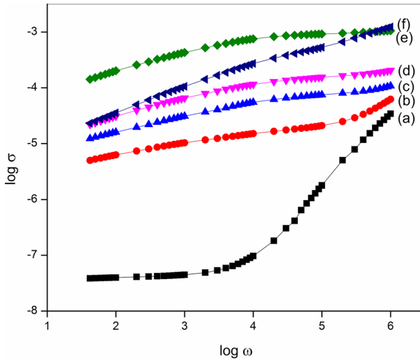
Fig. 6 Conductance spectra of (a) pure P(VdCl...), (b) 70 wt% P(VdCl...):30 wt% MgCl 2 , (c) 70 wt% P(VdCl...): 30 wt% MgCl 2 : 0.1 wt% SN, (d) 70 wt% P(VdCl...): 30 wt% MgCl 2 : 0.2 wt% SN, (e) 80 wt% P(VdCl...): 30 wt% MgCl 2 : 0.3 wt% SN, (f) 70 wt% P(VdCl...): 30 wt% MgCl 2 : 0.4 wt% SN
