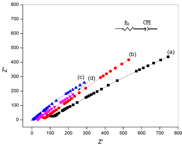
Fig. 5 Nyquist plot of (a) 70 wt% P(VdCl...): 30 wt% MgCl_2 : 0.1 wt% SN, (b) 70 wt% P(VdCl...): 30 wt% MgCl_2 : 0.2 wt% SN, (c) 70 wt% P(VdCl...): 30 wt% MgCl_2 : 0.3 wt% SN and (d) 70 wt% P(VdCl...): 30 wt% MgCl_2 : 0.4 wt% SN
