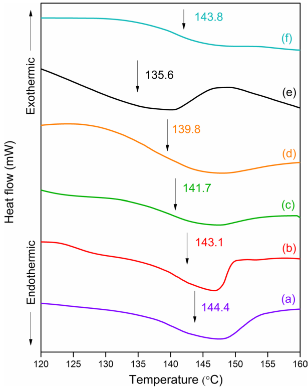
Fig. 3 DSC curves of (a) pure P(VdCl...), (b) 70 wt% P(VdCl...):30 wt% MgCl 2 , (c) 70 wt% P(VdCl...): 30 wt% MgCl 2 ; 0.1 wt% SN, (d) 70 wt% P(VdCl...): 30 wt% MgCl 2 ; 0.2 wt% SN, (e) 70 wt% P(VdCl...): 30 wt% MgCl 2 ; 0.3 wt% SN, (f) 70 wt% P(VdCl...): 30 wt% MgCl 2 ; 0.4 wt% SN
